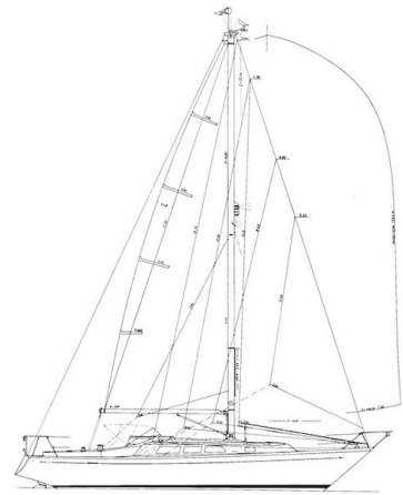
Segelplan
